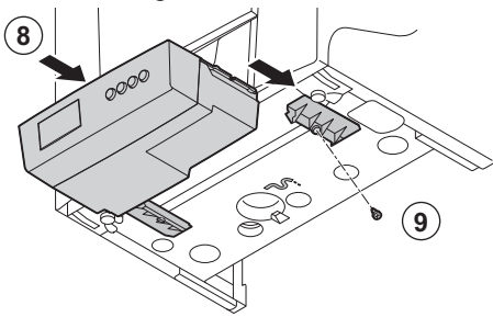
Abb.21 Anbringen der Control Box
