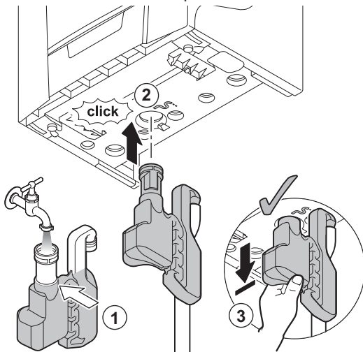
Abb.31 Befüllen des Siphons
