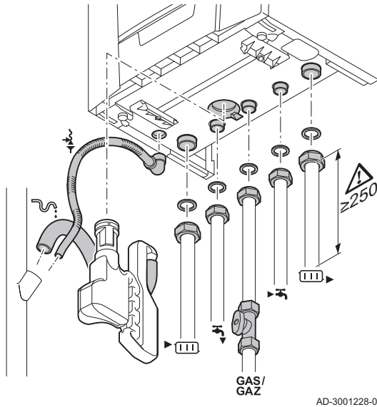
Abb.17 Verbinden
