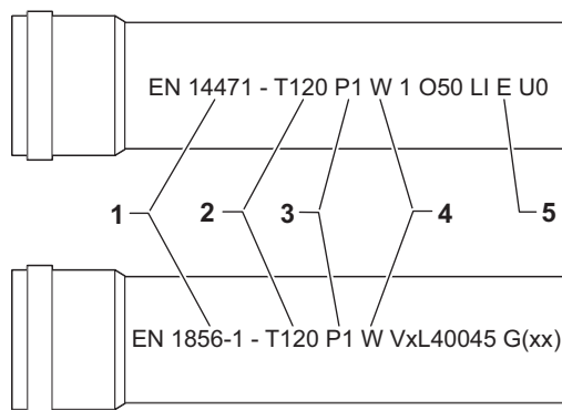
Abb.5 Probestück
