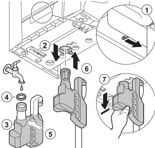
Abb.58 Reinigung des Siphons
