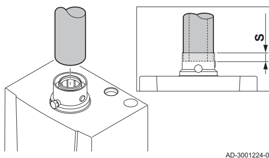
Abb.18 Anschluss des Abgasstutzens und der Luftzufuhr
