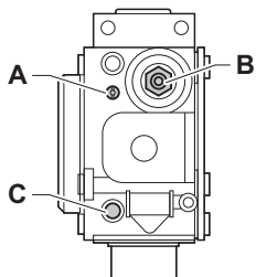
Abb.33 Gasventilbaugruppe
