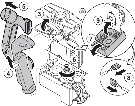
Abb.61 Ausbau
