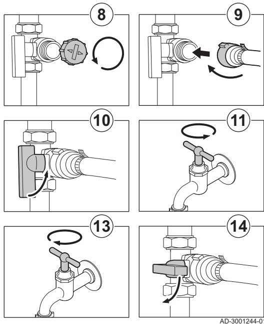
Abb.72 Nachfüllen der Anlage
