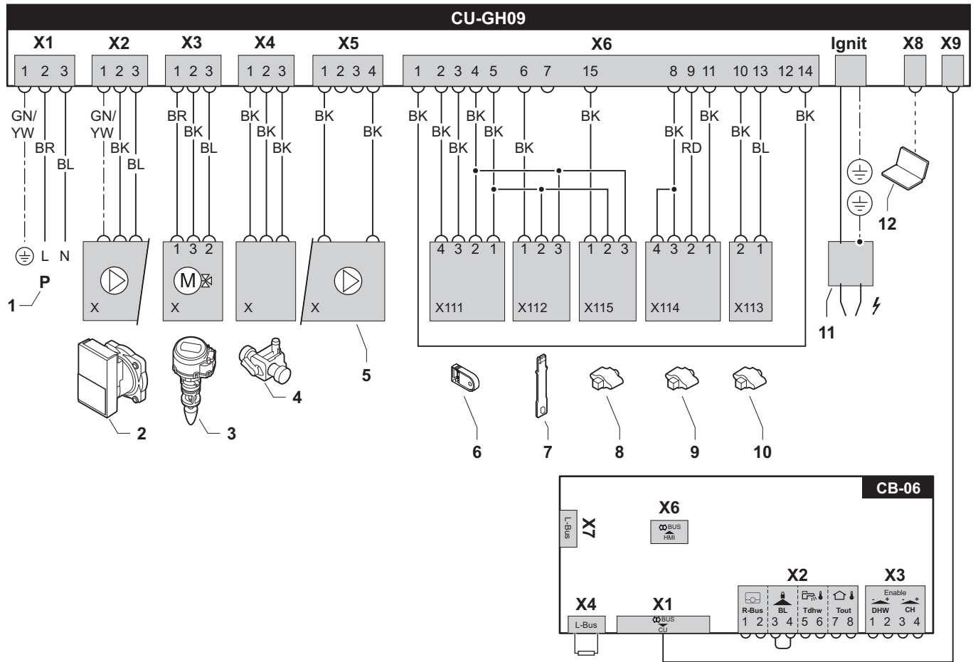
Abb.78 Elektrischer Schaltplan
