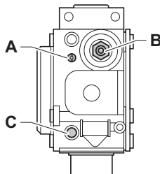
Abb.37 Gasventilbaugruppe
