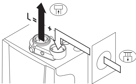
Abb.12 Unterschiedliche Druckbereiche
