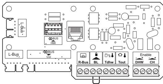
Abb.22 Standard-Regelungsleiterplatte (CB-06)
