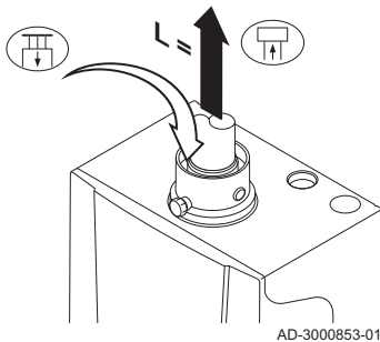
Abb.9 Raumluftabhängige Version (concentrisch)
