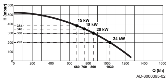
Abb.80 Tzerra Ace 28C
