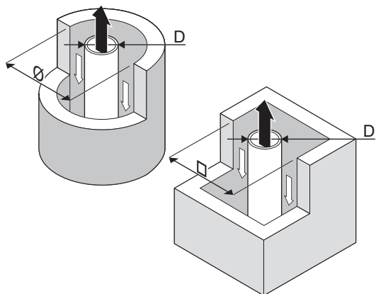
Abb.4 Mindestabmessungen des Schachts oder Kanals
