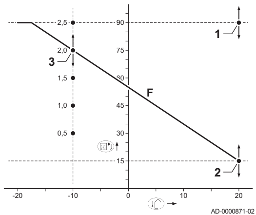
Abb.54 Interne Heizkennlinie
