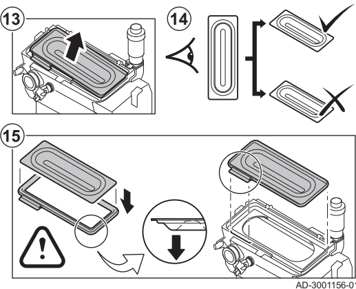
Abb.62 Kontrolle
