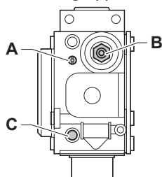
Abb.39 Gasventilbaugruppe
