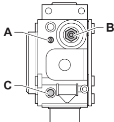
Abb.32 Prüfföffnungen der Gasventilbaugruppe
