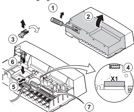
Abb.20 Zugang zu den Anschlüssen
