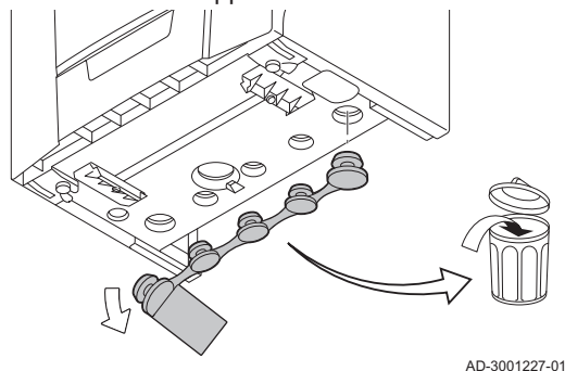
Abb.16 Schutzkappen entfernen
