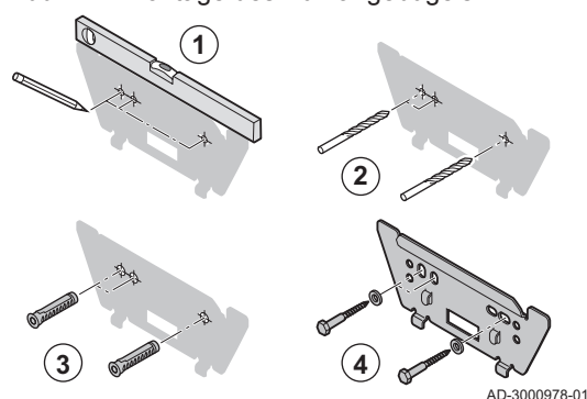
Abb.15 Montage des Heizkessels
