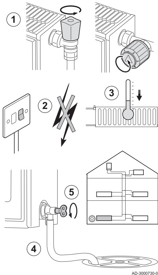
Abb.76 Entleeren der Anlage
