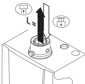
Abb.13 CLV-Überdrucksystem
