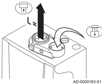
Abb.9 Raumluftabhängige Version (concentrisch)
