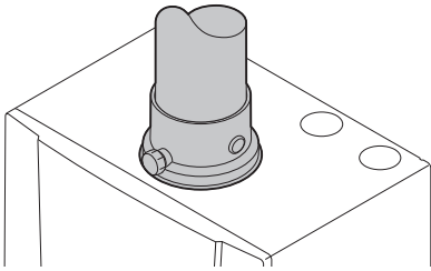
Abb.56 Prüfung des Abgasstutzens und der Luftzufuhr
