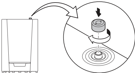
Abb.57 Überprüfung des automatischen Schnellentlüfters
